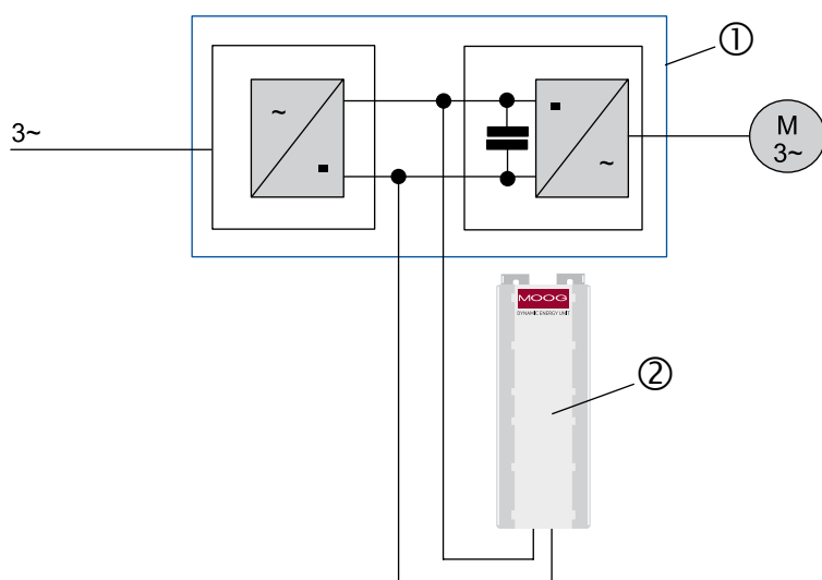
Fig. 5: Anschlussschema
