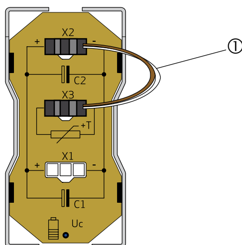
Fig. 14: Erweiterungsmodul entladen (Gehäuseoberseite)
