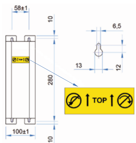
Fig. 3: Bohrschablone
