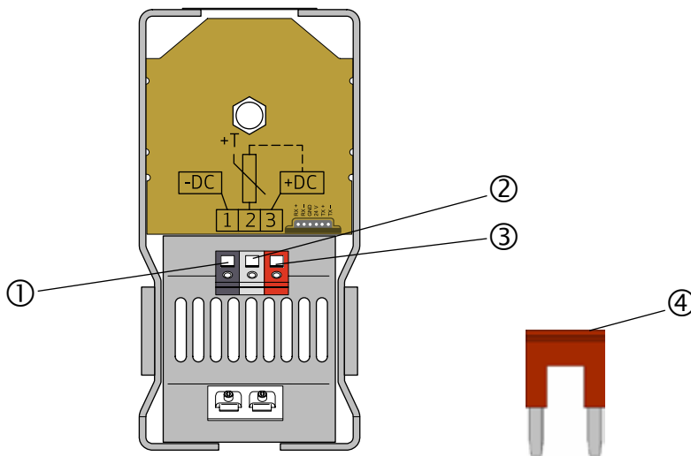
Fig. 6: Anschlussklemmen, Gehäuseunterseite
