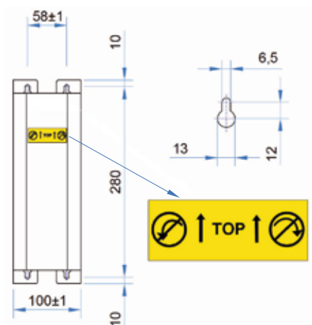
Fig. 3: Bohrschablone
