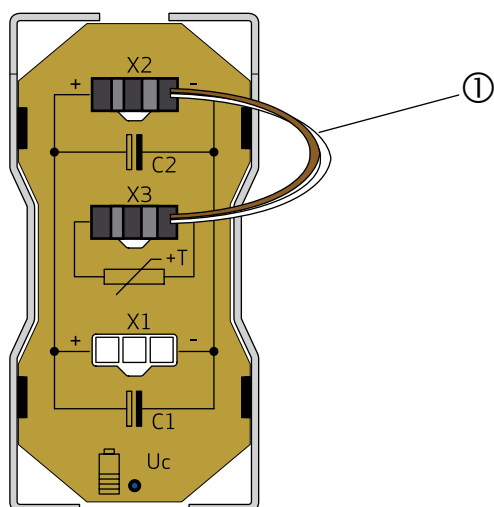
Fig. 15: Erweiterungsmodul 2 entladen (Gehäuseoberseite)
