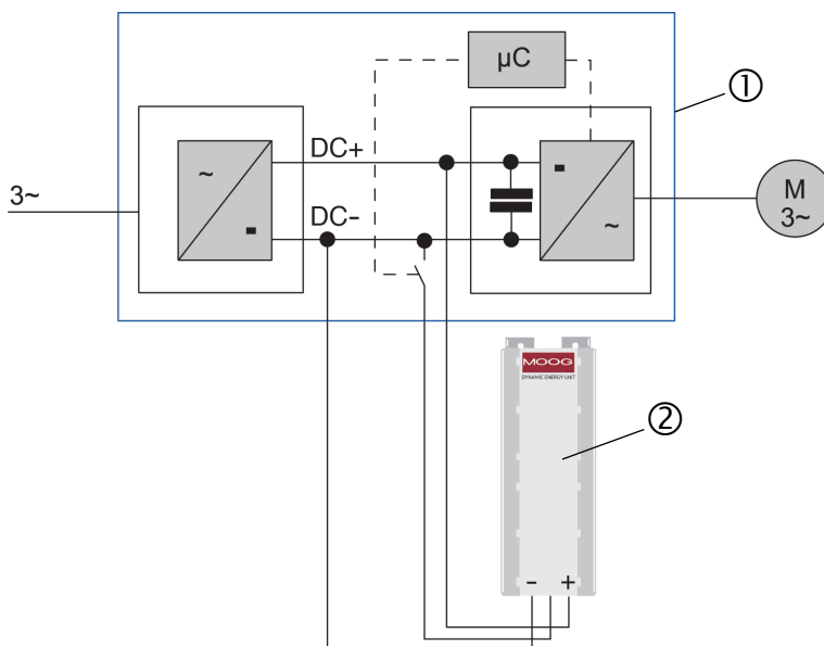
Fig. 5: Anschlussschema
