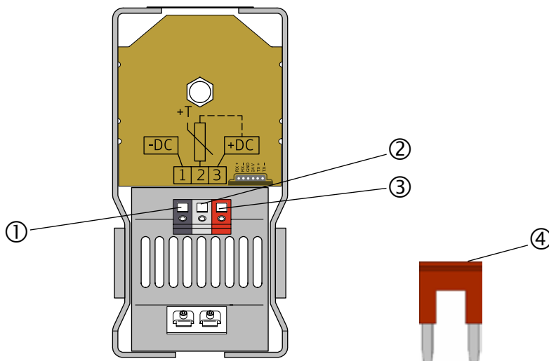
Fig. 10: DEU-ST entladen
