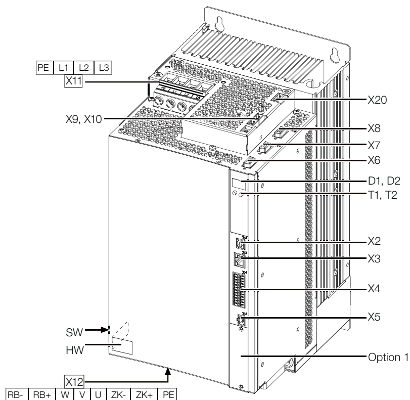
Bild 4.6 Lageplan BG5 (hier: Gehäusevariante Wandmontage)
