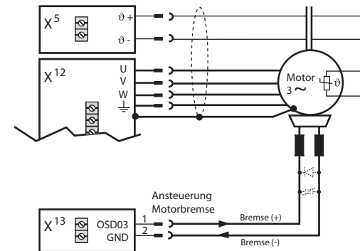
Bild 4.19 Anschluss des Motors bei BG1 bis BG4
