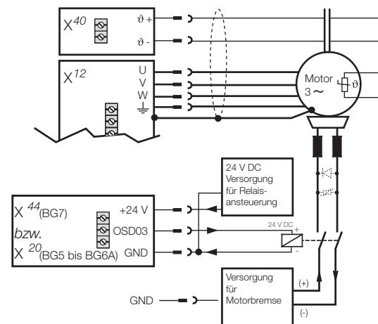
Bild 4.20 Anschluss des Motors bei BG5 bis BG7
