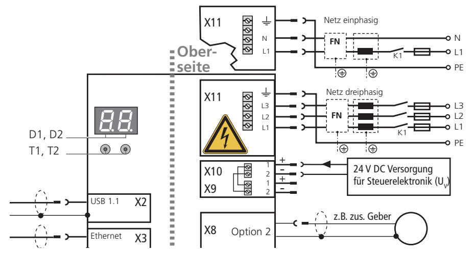
Bild 4.15 Anschlussbeispiel Steuer- /Netzversorgung für BG1 bis BG4
