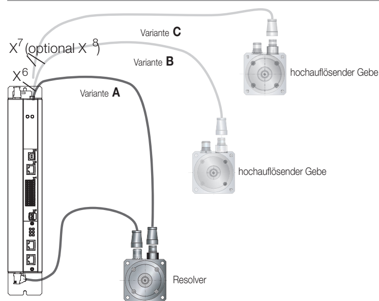
Bild 4.18 Zuordnung Motor-/Geberleitung
