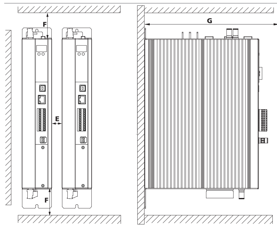
Bild 3.1 Montageabstände bei Luftkühlung, schematische Darstellung für BG1 bis BG6A
