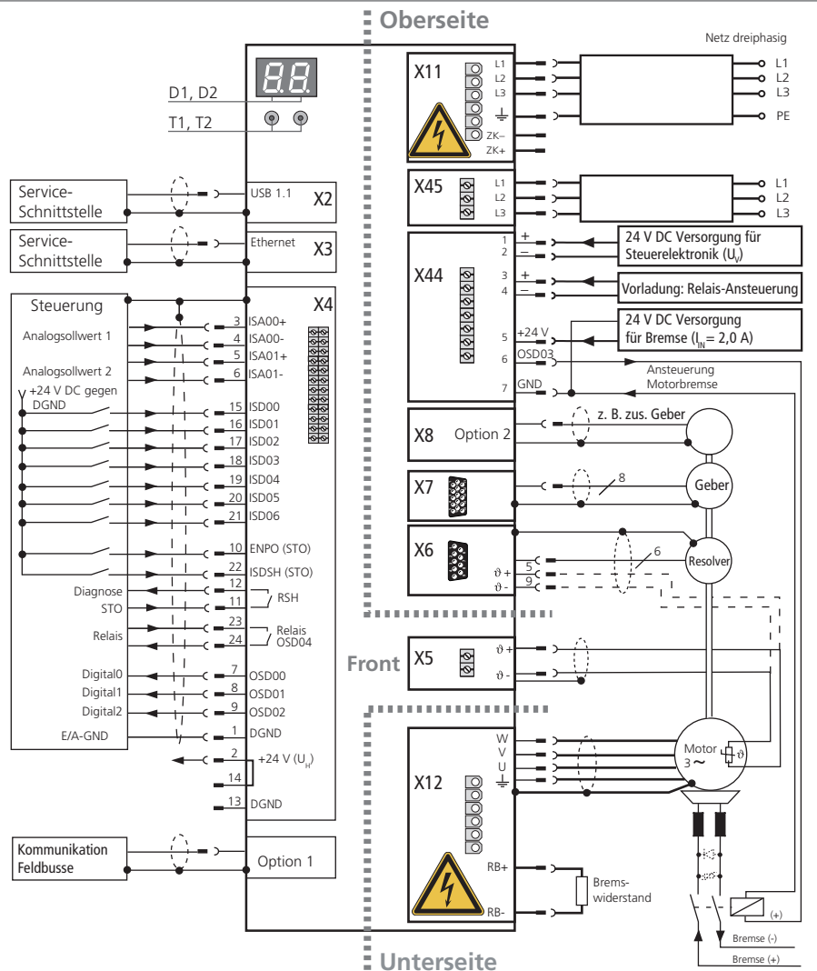
Bild 4.10 Anschlussplan BG7
