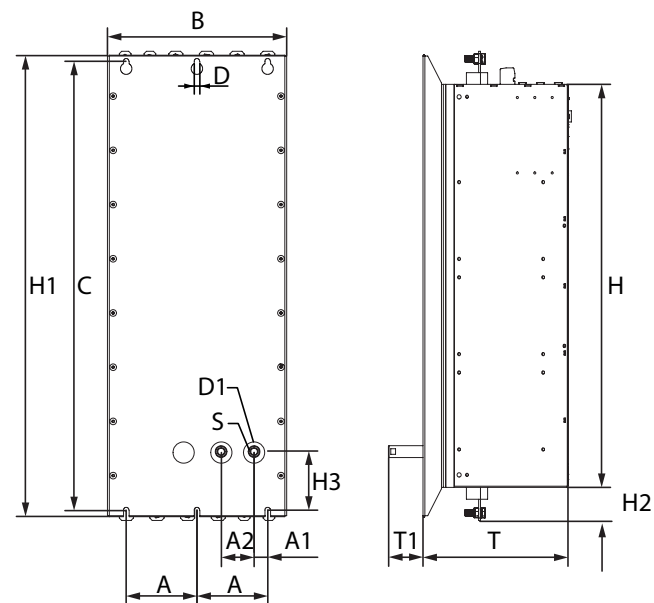
Bild 3.5 Maßzeichnung Gehäuse mit Flüssigkeitskühlung, schematische Darstellung für BG7
