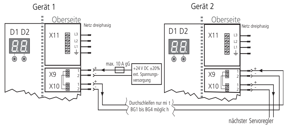
Bild 4.14 Anschluss Steuerversorgung BG1 bis BG6A
