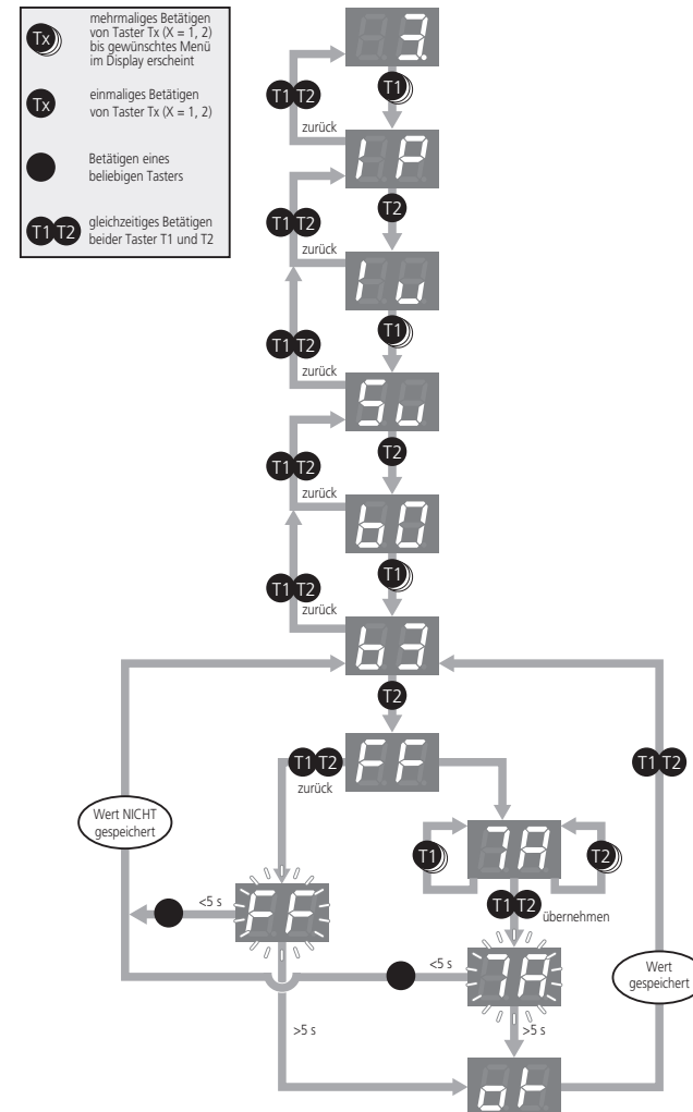
Bild 5.3 Beispielkonfiguration der Subnetzmaske
