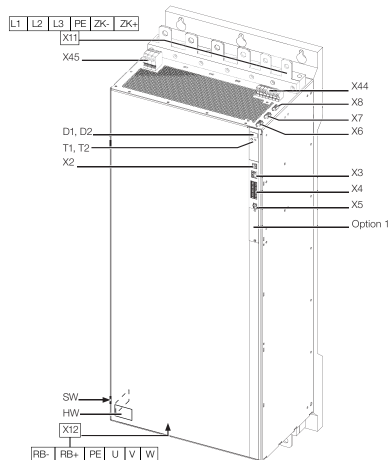
Bild 4.9 Lageplan BG7 (ohne Schirmbleche und Klemmenabdeckungen an X11 und X12)
