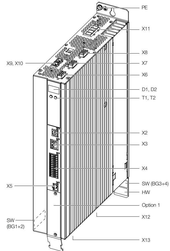
Bild 4.4 Lageplan BG1 bis BG4 (hier: BG1)
