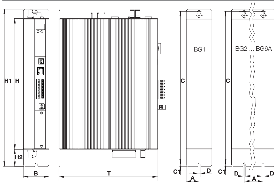
Bild 3.2 Maßzeichnung Gehäuse mit Luftkühlung, schematische Darstellung für BG1 bis BG6A
