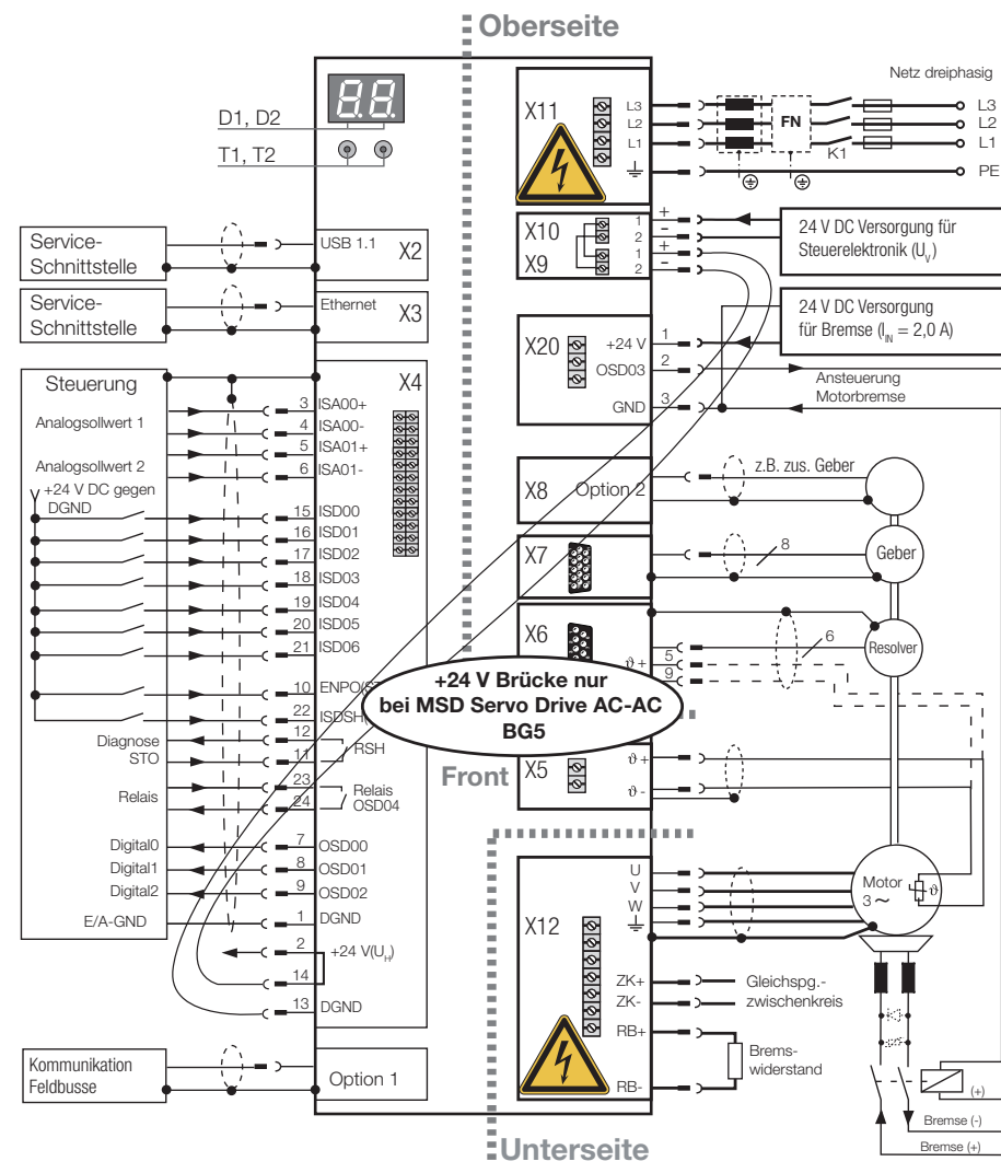
Bild 4.8 Anschlussplan BG5 bis BG6A
