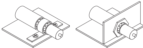
Bild 4.1 Schirmanschluss RICHTIG
