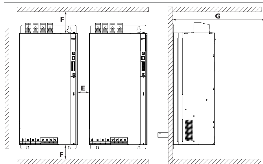
Bild 3.3 Montageabstände bei Flüssigkeitskühlung, schematische Darstellung für BG3 bis BG7
