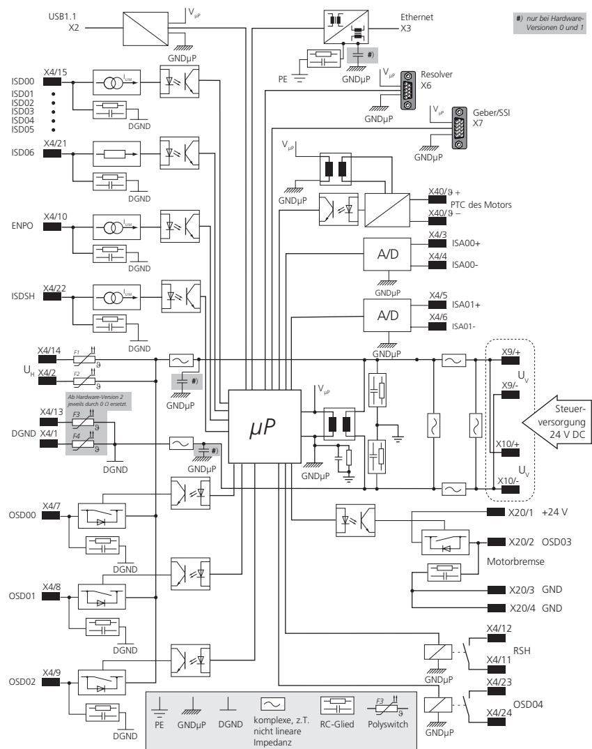
Bild 4.12 Potenzialtrennkonzzept für BG1 bis BG4
