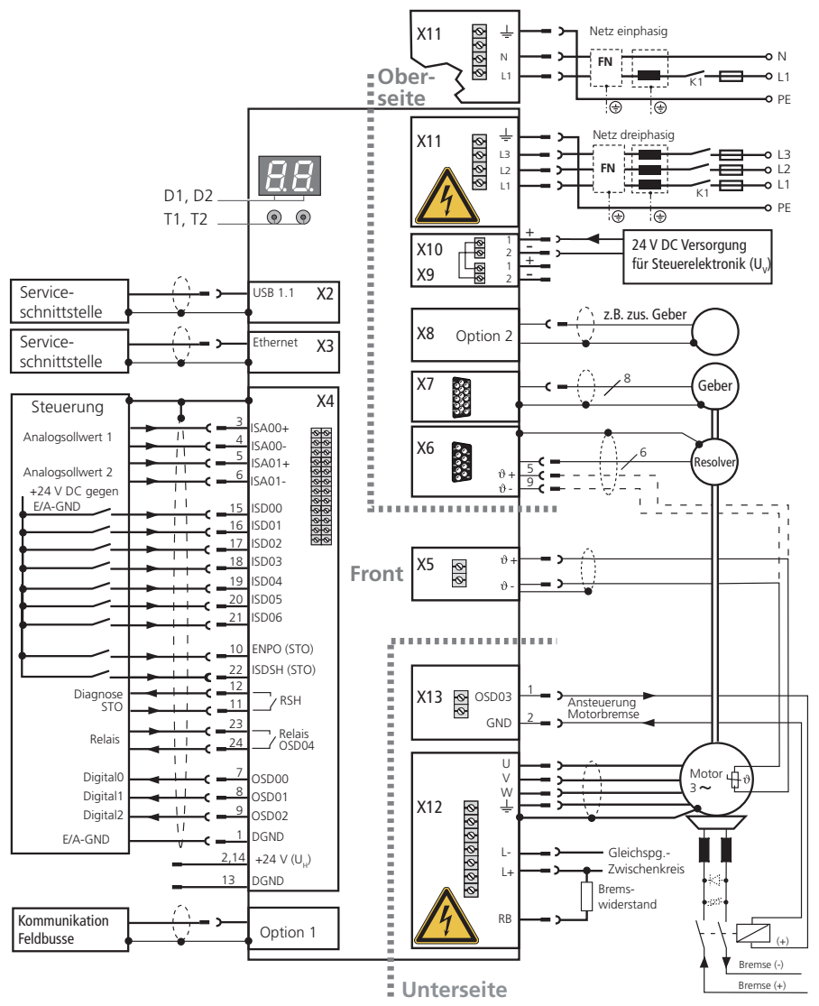
Bild 4.5 Anschlussplan BG1 bis BG4
