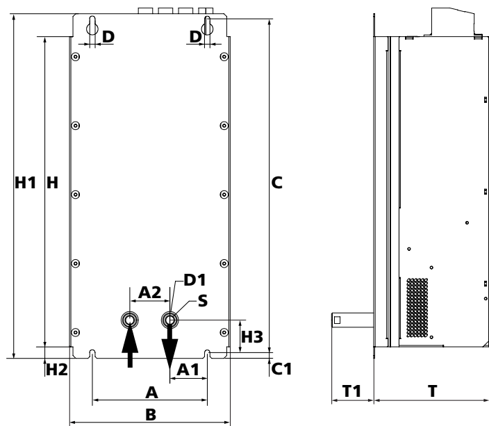
Bild 3.4 Maßzeichnung Gehäuse mit Flüssigkeitskühlung, schematische Darstellung für BG3 bis BG6A
