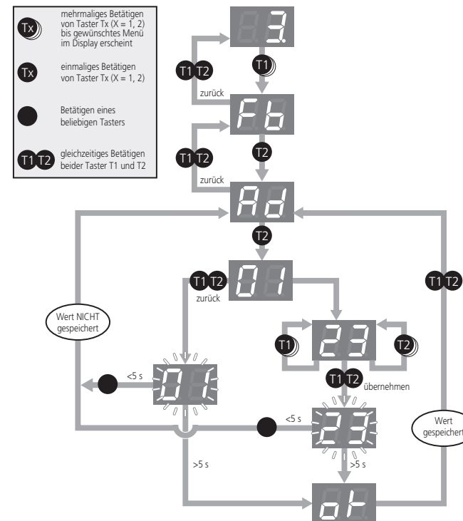
Bild 5.4 Beispielkonfiguration der Feldbus-Adresse
