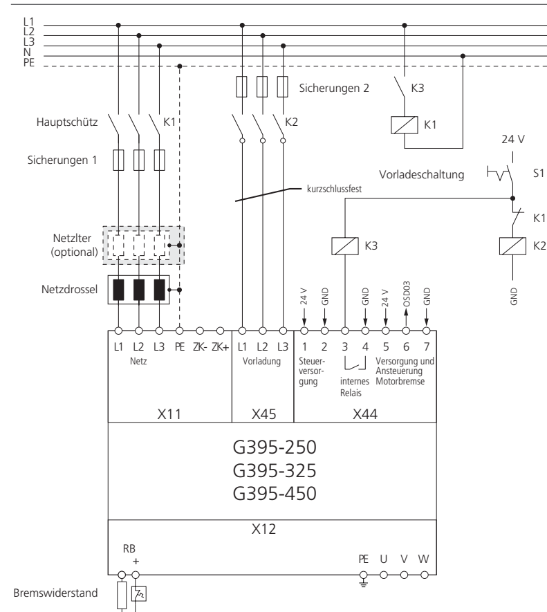
Bild 4.17 Anschluss Vorladung, Steuer- und Netzversorgung 3 x 230/400/460/480 V für BG7
