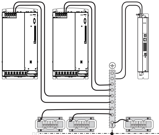
Bild 4.11 Sternförmige Verlegung des Schutzleiters
