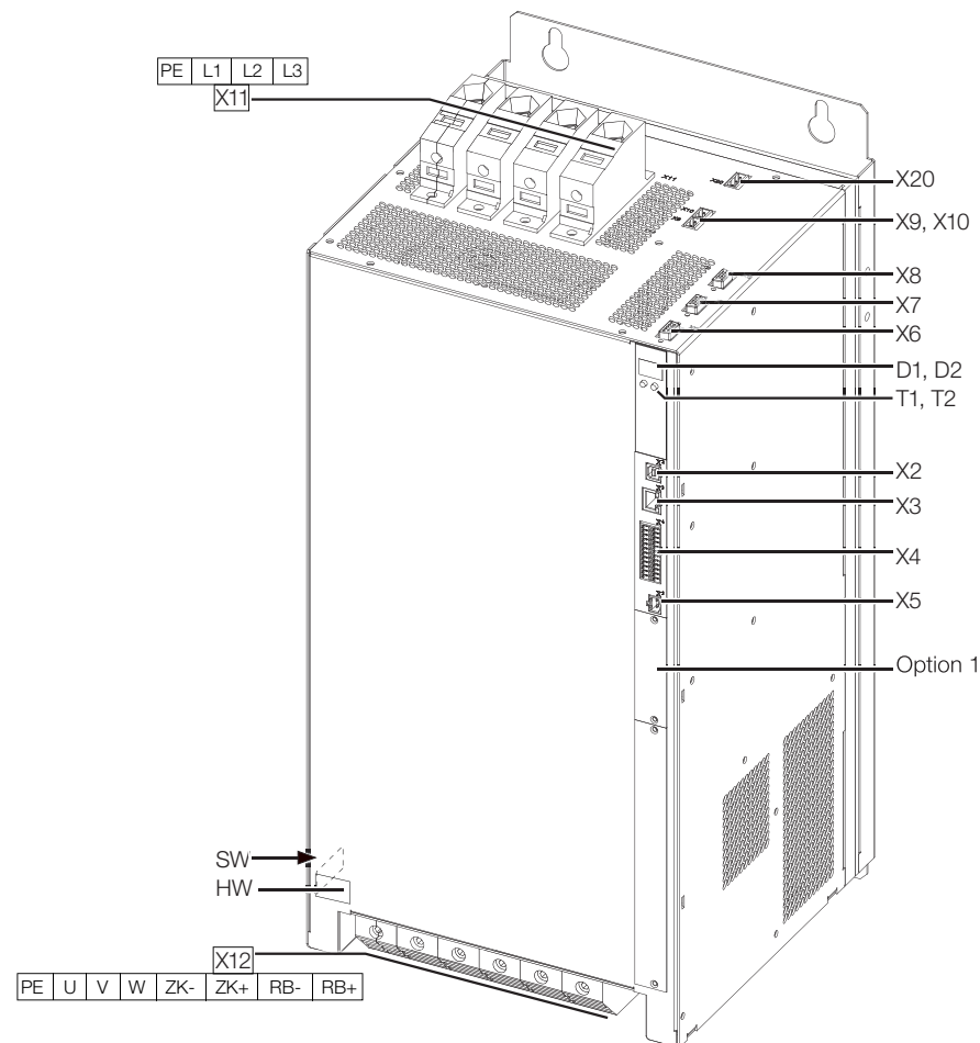
Bild 4.7 Lageplan BG6 und BG6A (hier: BG6A, Gehäusevariante Flüssigkeitskühlung)
