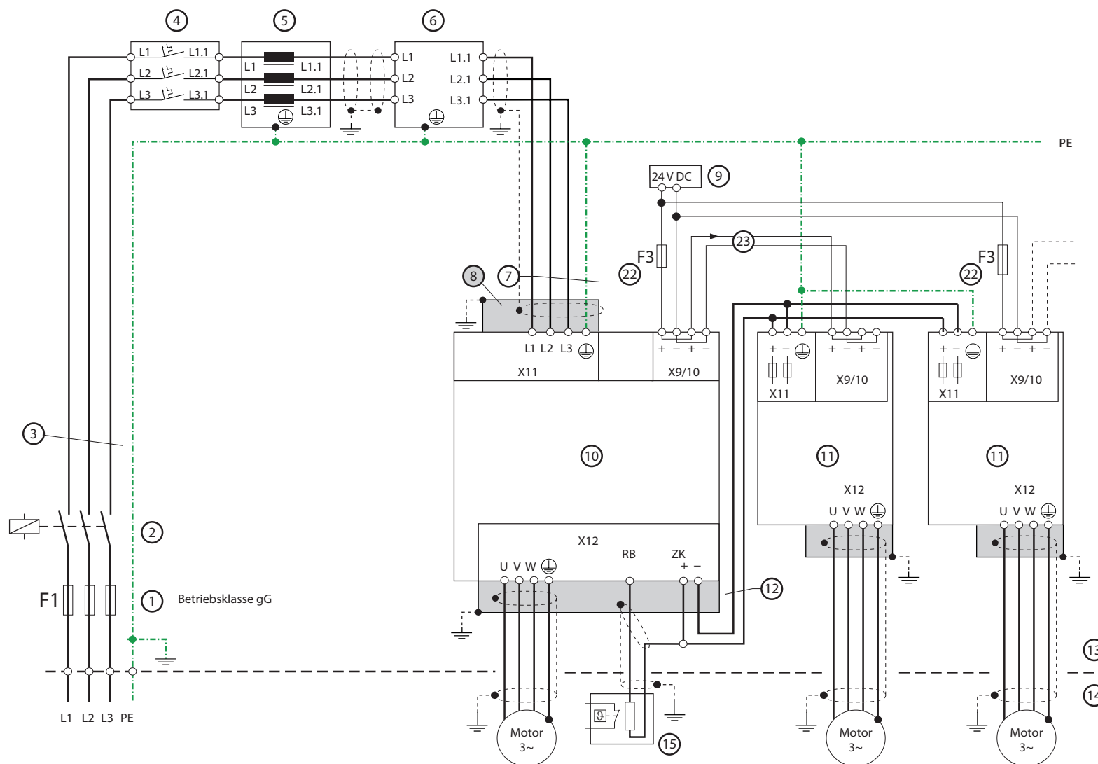
Bild 8.1 Übersicht Anschlussplan für Betrieb mit Versorgung durch AC-AC Servoregler (BG1 bis BG5)
