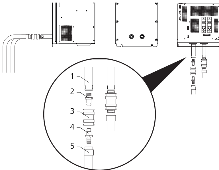
Bild 3.19 Anschluss Kühlkreislauf beispielhaft BG6A und BG7
