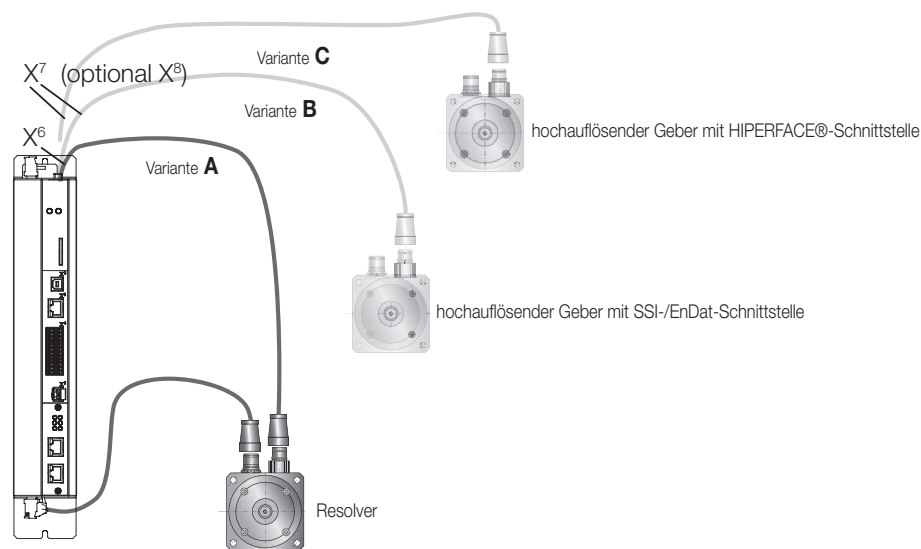
Bild 4.18 Zuordnung Motor-/Geberleitung
