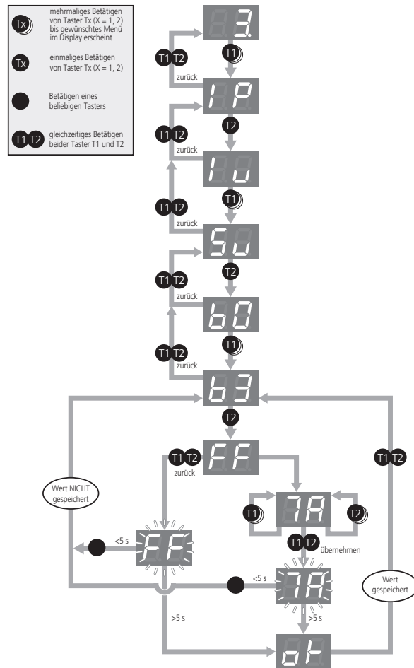
Bild 5.2 Beispielkonfiguration der Subnetzmaske
