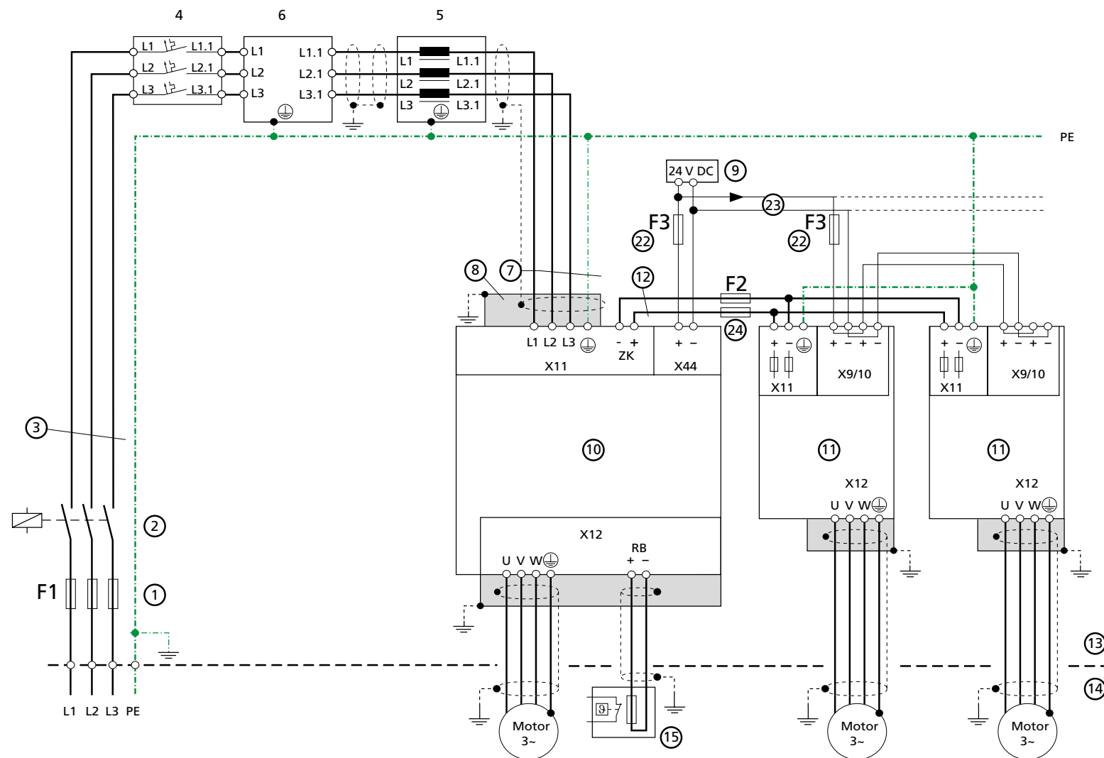
Bild 8.3 Übersicht Anschlussplan für Betrieb mit Versorgung durch AC-AC Servoregler (BG7)
