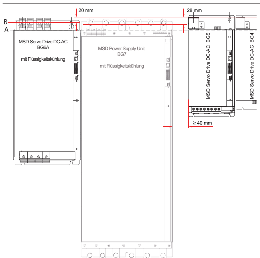
Bild 3.14 Ausrichtung DC-AC Servoregler an Versorgungseinheit BG7 (Beispiel)
