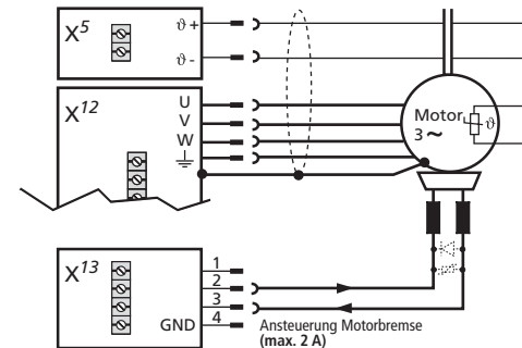
Bild 4.19 Anschluss des Motors bei BG1 bis BG4 (Motorbremse bis 2 A)
