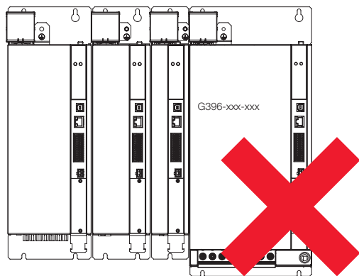
Bild 3.6 Beispiel einer nicht zulässigen Anordnung: Anreihung von DC-AC Servoreglern mit aufsteigender Baugröße
