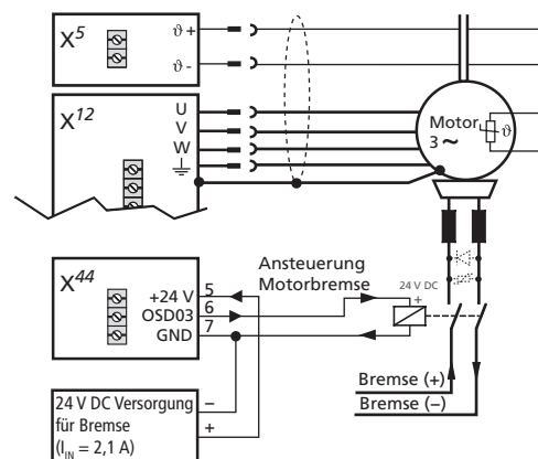
Bild 4.22 Anschluss des Motors für G397-250 bis G397-450 (BG7)
