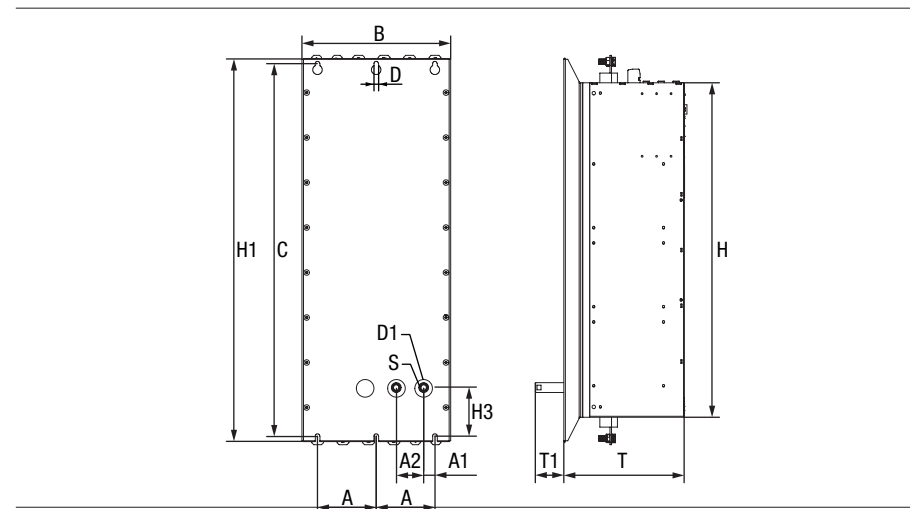
Bild 3.16 Maßzeichnung Gehäusevariante Flüssigkeitskühlung beispielhaft BG7
