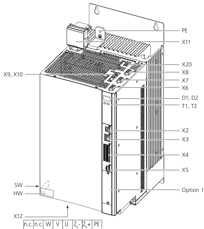
Bild 4.6 Lageplan G393-045/G397-053 bis G393-072/G397-084 (BG5, ohne Schirmbleche)
