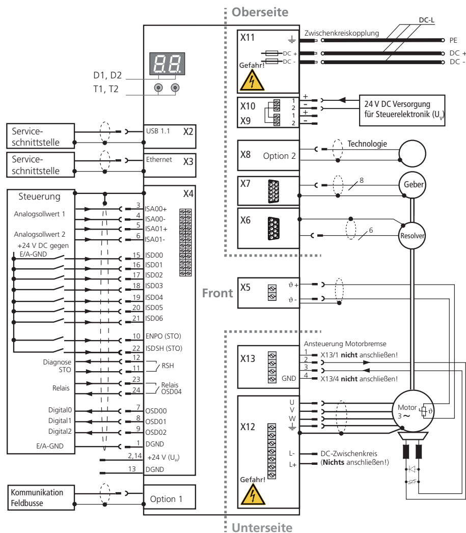
Bild 4.5 Anschlussplan G393-004 (BG1) bis G393-032/G397-035 (BG4)
