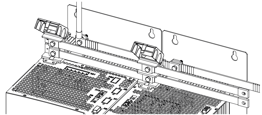
Bild 4.15 Detail: Anschluss DC-Leistungsversorgung BG5
