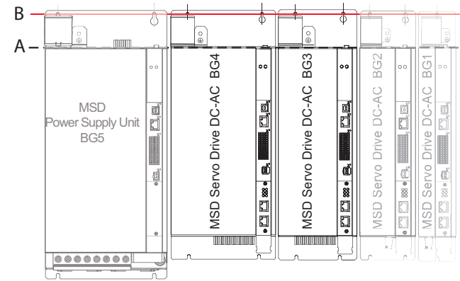
Bild 3.12 Ausrichtung DC-AC Servoregler an Versorgungseinheit BG5 (Beispiel)
