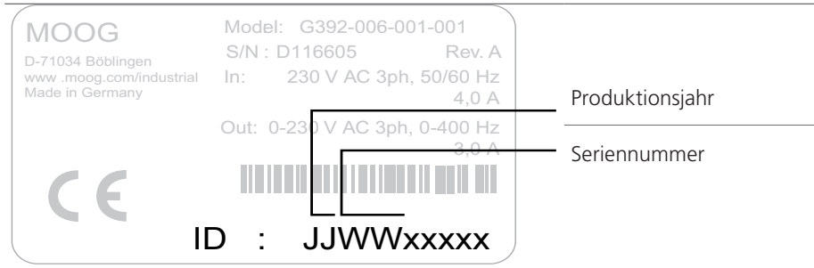
Bild 1.1 Typenschild Hardware DC-AC Servoregler
