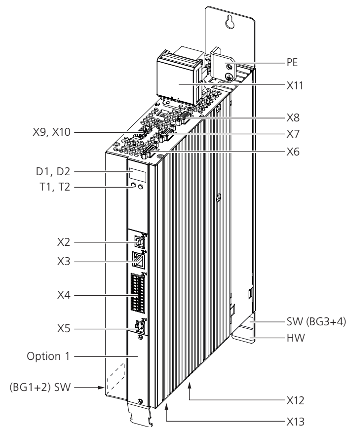
Bild 4.4 Lageplan G393-004 (BG1) bis G393-032/G397-035 (BG4) (beispielhaft G393-004 BG1)
