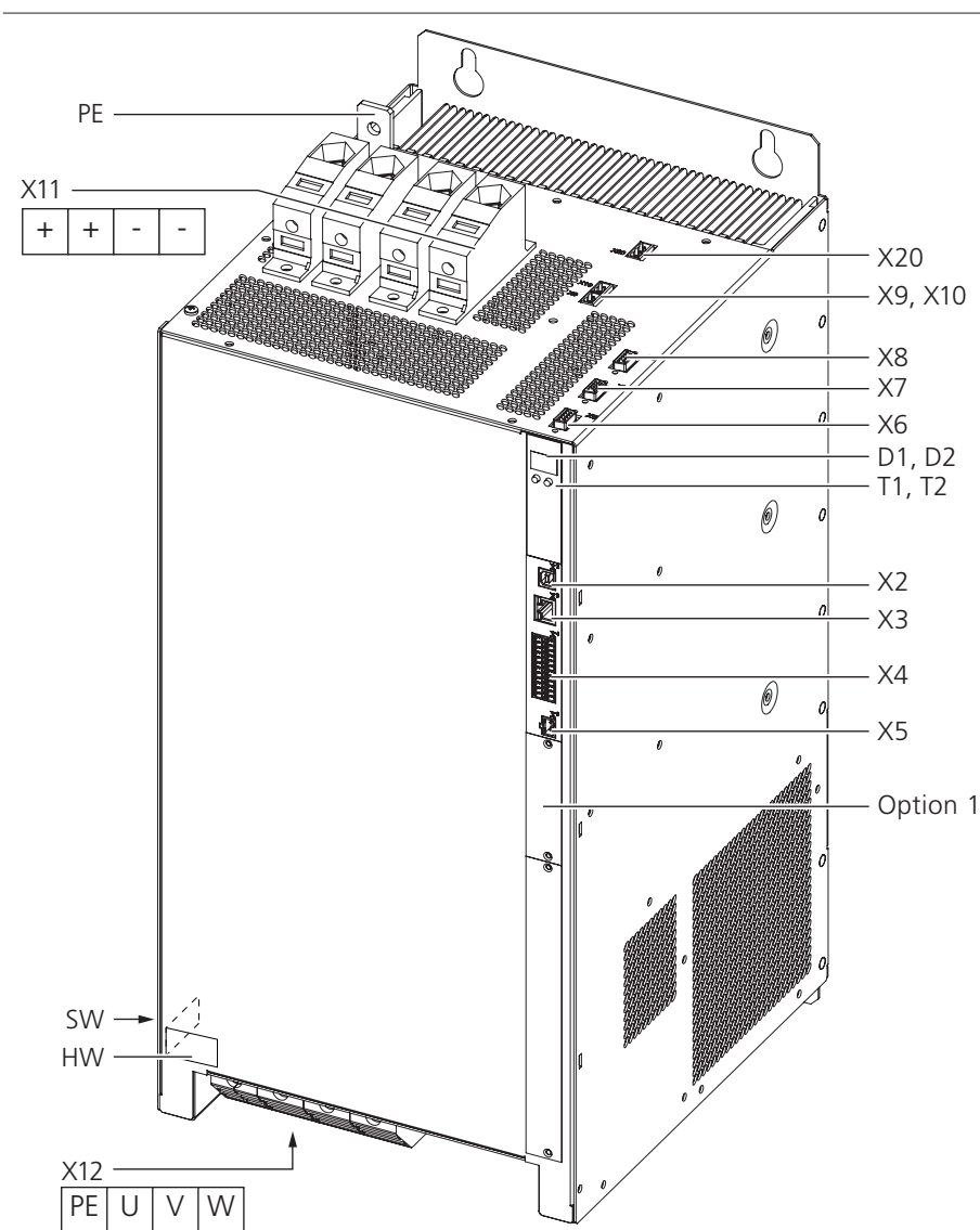
Bild 4.7 Lageplan G393-090/G397-110 bis G393-170/G397-210 (BG6A, ohne Schirmbleche)
