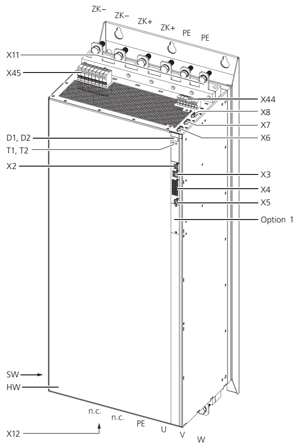
Bild 4.9 Lageplan G393-250 bis G393-450 (BG7, ohne Schirmbleche)
