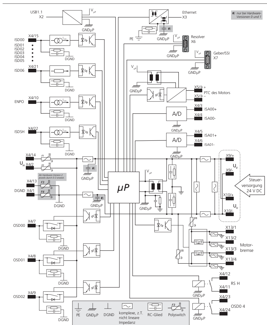
Bild 4.11 Potenzialtrennkonzzept BG1 bis BG4
