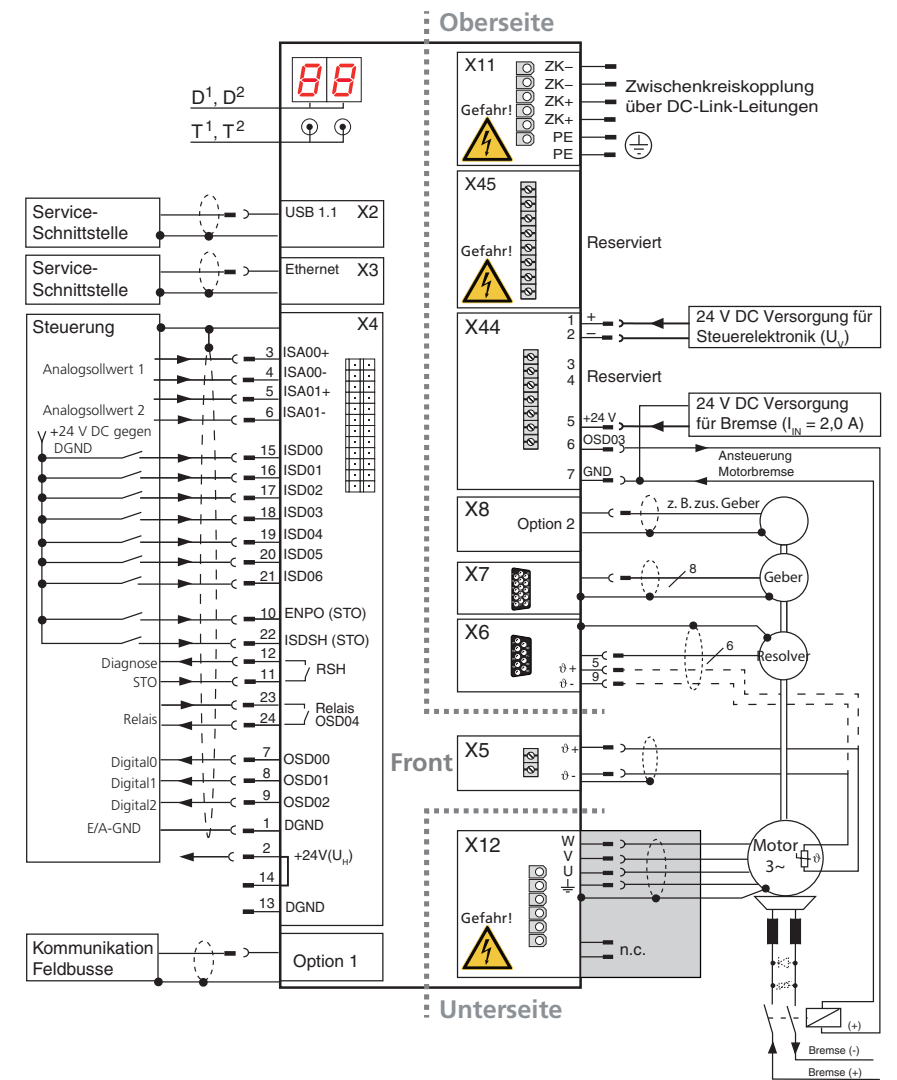
Bild 4.10 Anschlussplan G393-250 bis G393-450 (BG7)
