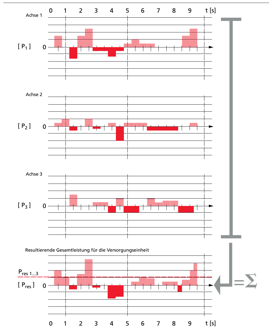
Bild 9.3 Zeit-/Leistungsdiagramm mit Versorgungseinheit
