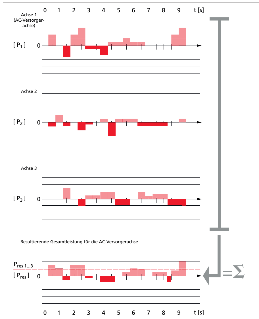
Bild 9.4 Zeit-/Leistungsdiagramm mit AC-AC Servoregler als Versorgung
