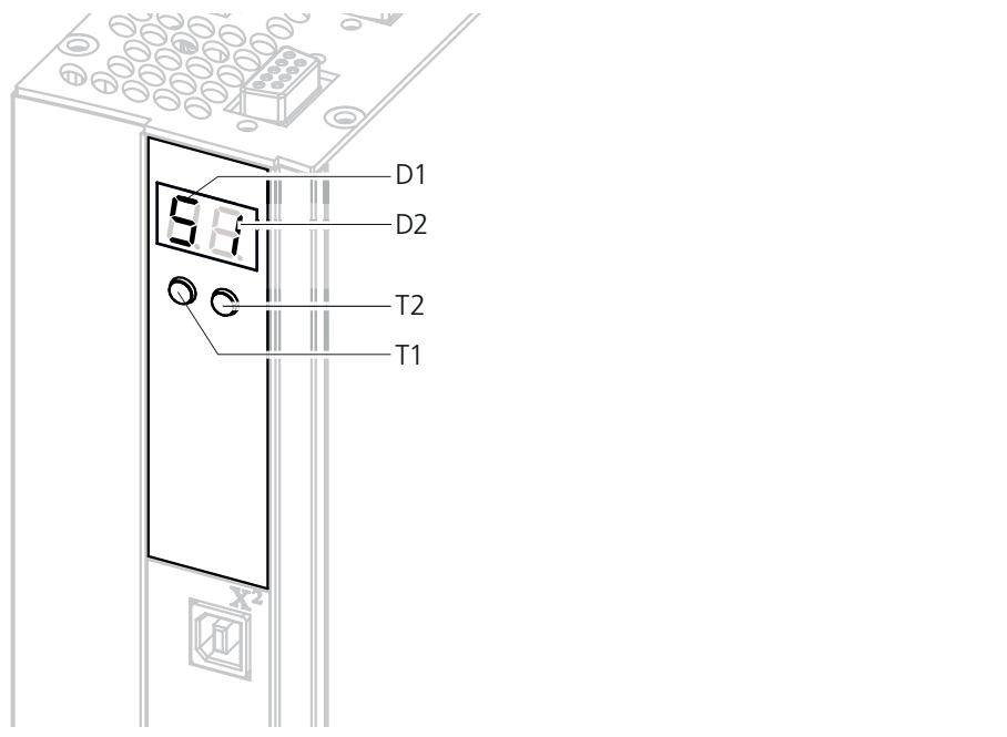
Bild 5.1 Integrierte Bedieneinheit
