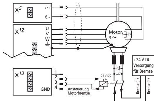
Bild 4.20 Anschluss des Motors bei BG1 bis BG4 (Motorbremse ab 2 A)
