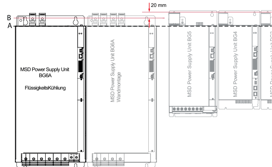
Bild 3.13 Ausrichtung DC-AC Servoregler an Versorgungseinheit BG6A (Beispiel)
