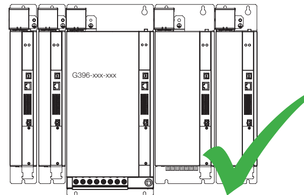
Bild 3.5 Beispiel einer zulässigen Anordnung: Anreihung von DC-AC Servoreglern mit gleicher bzw. absteigender Baugröße beidseitig der Versorgungseinheit
