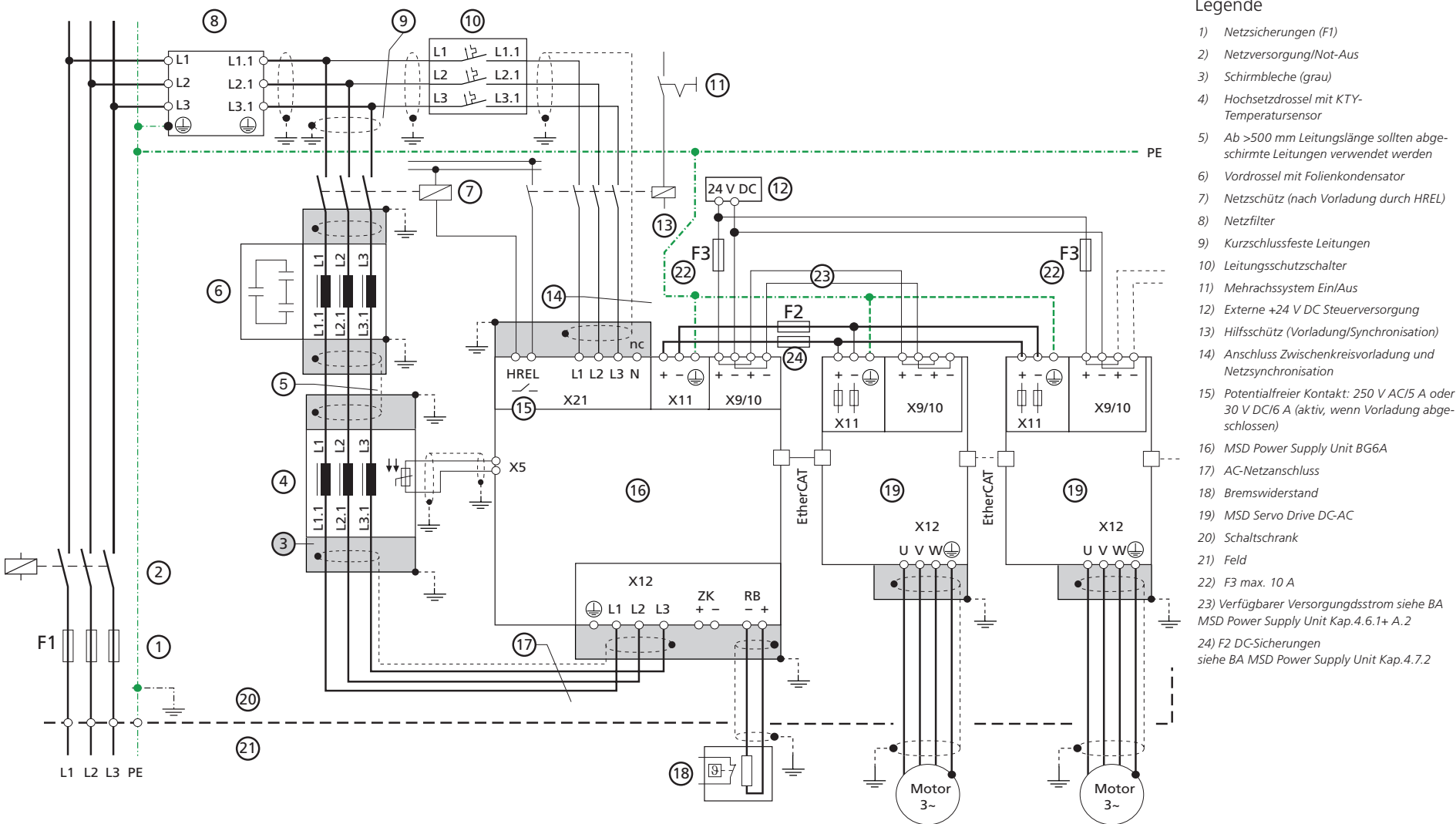
Bild 4.17 Anschluss Leistungs- und Steuerversorgung sowie Schutzleiter im Achsverbund (Beispiel)
