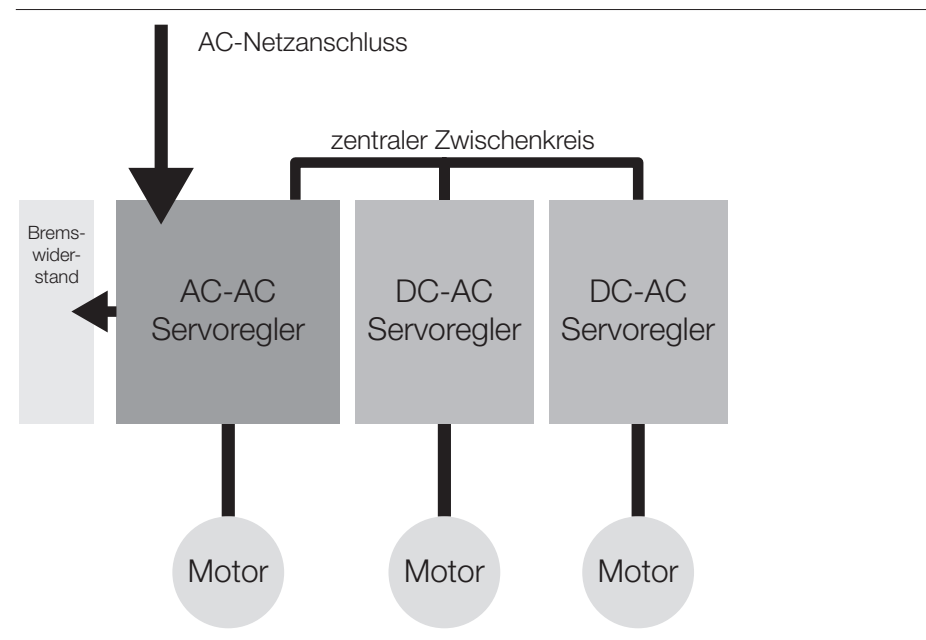
Bild 9.2 Blocksaltbild eines Mehrachssystems mit AC-AC Servoregler als Versorgung
