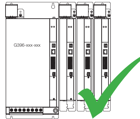
Bild 3.4 Beispiel einer zulässigen Anordnung: Anreihung von DC-AC Servoreglern mit gleicher Baugröße an einer Seite der Versorgungseinheit
