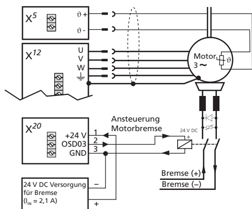
Bild 4.21 Anschluss des Motors für G393-045/G397-053 (BG5) bis G393-170/G397-210 (BG6A)
