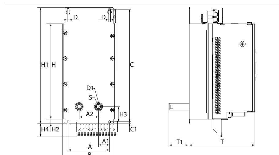
Bild 3.15 Maßzeichnung Gehäusevariante Flüssigkeitskühlung beispielhaft BG5
