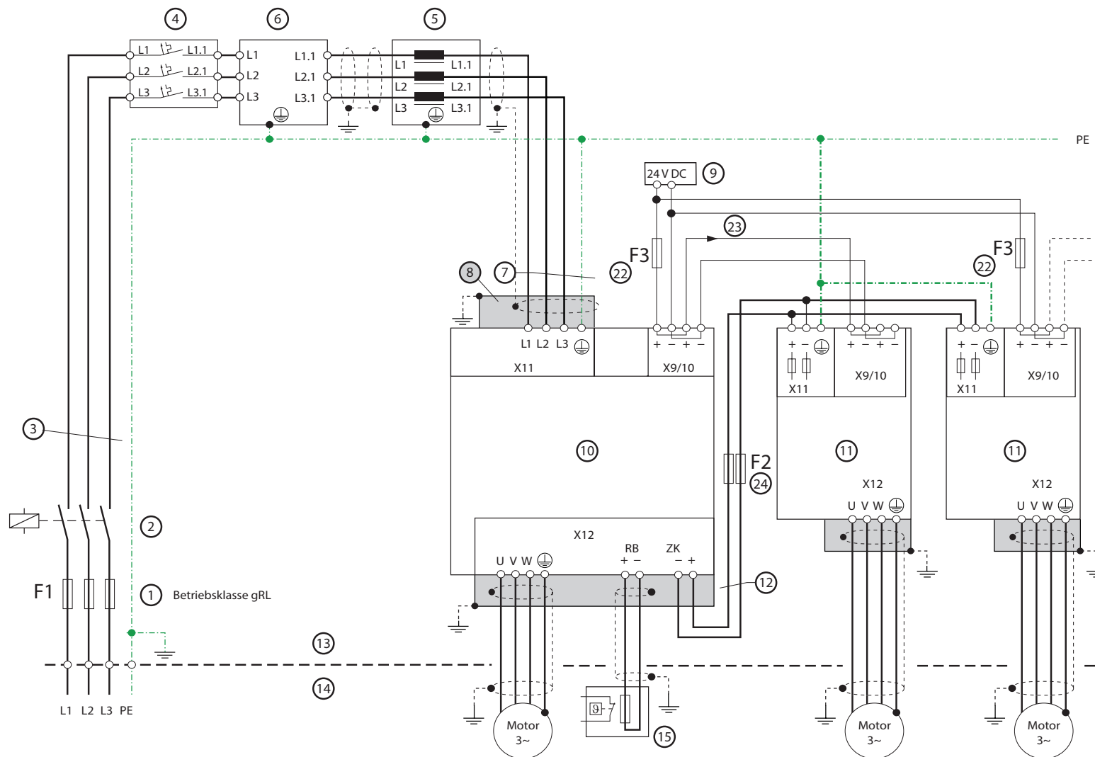
Bild 8.2 Übersicht Anschlussplan für Betrieb mit Versorgung durch AC-AC Servoregler (BG6 bis BG6A)
