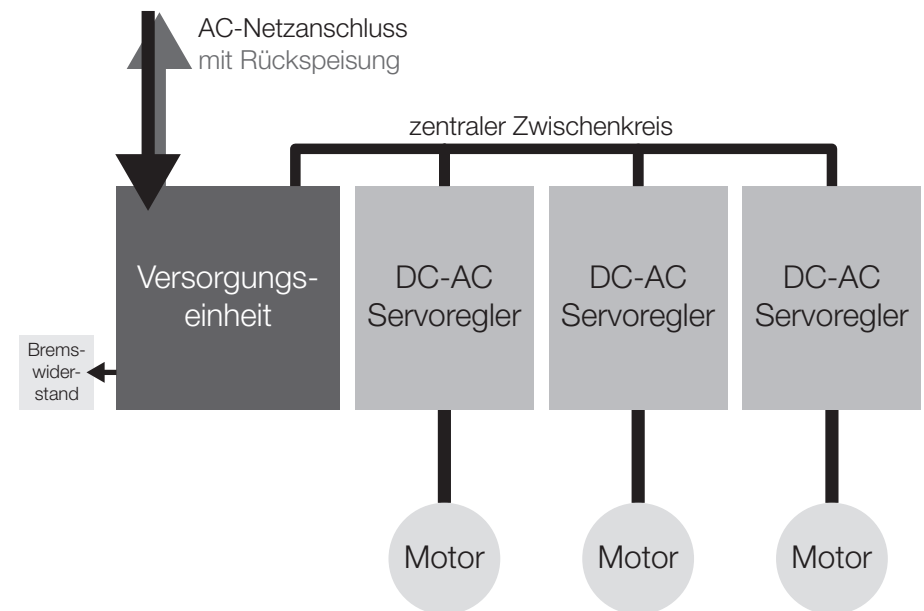
Bild 9.1 Blockschaltbild eines Mehrachssystems mit Versorgungseinheit und Netzurückspeisung
