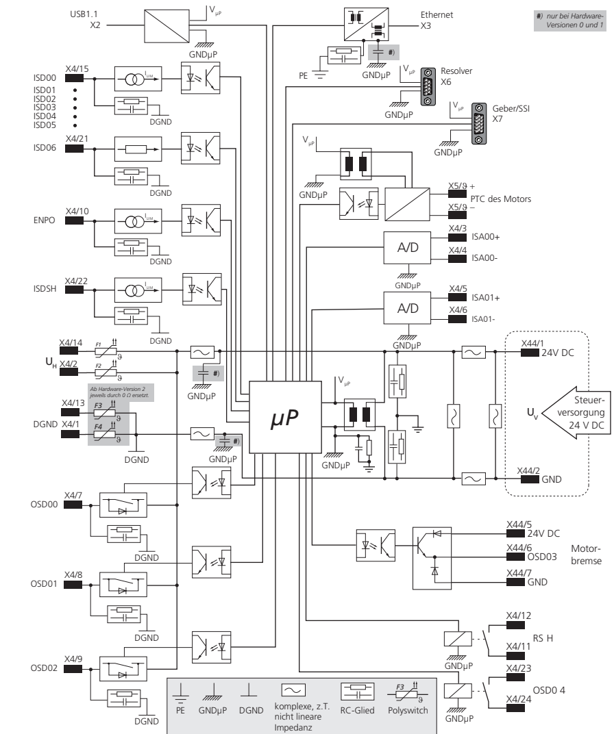
Bild 4.13 Potenzialtrennkonzzept BG7
