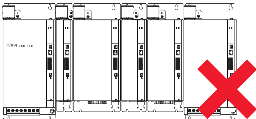
Bild 3.7 Beispiel einer nicht zulässigen Anordnung: Anreihung von DC-AC Servoreglern mit auf- und absteigenden Baugrößen
