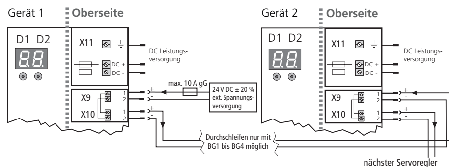
Bild 4.14 Anschluss Steuerversorgung
