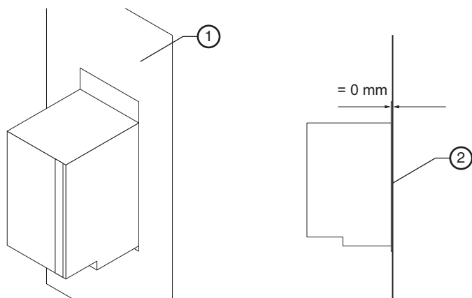
Bild 3.2 Montage DC-AC Servoregler RICHTIG
