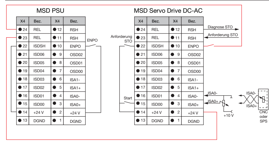
Bild 10.1 Verriegelung MSD Mehrachssystem (Beispiel)
