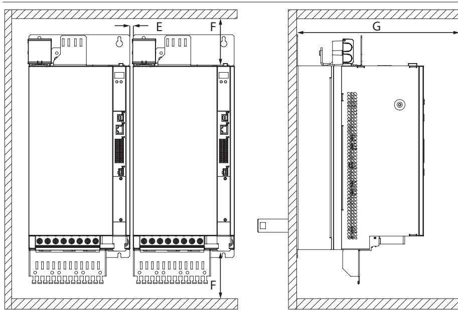
Bild 3.17 Montageabstand Gehäusevariante Flüssigkeitskühlung beispielhaft BG5
