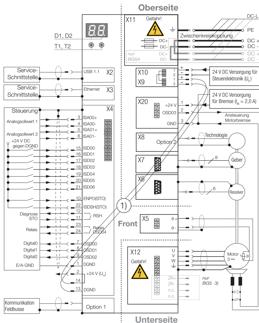
Bild 4.8 Anschlussplan G393-045/G397-053 (BG5) bis G393-170/G397-210 (BG6A)
